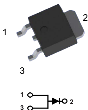
TO-252 MUR550D-S
